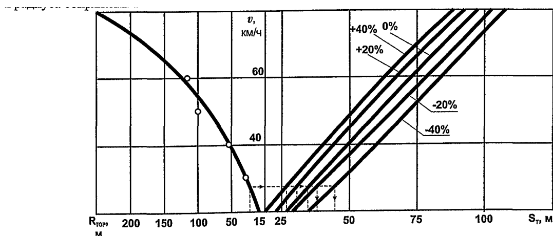
Рисунок 6.5 – График уменьшения длины полосы торможения при различных продольных уклонах в зависимости от радиуса сопряжения съездов
