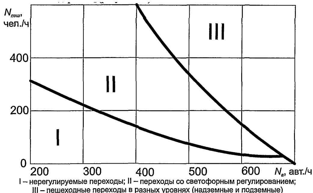
Рисунок 6.1 – Области применения пешеходных переходов различных типов
