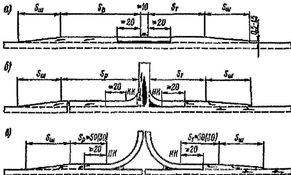
Рисунок 6.7 – Схемы переходно-скоростных полос
