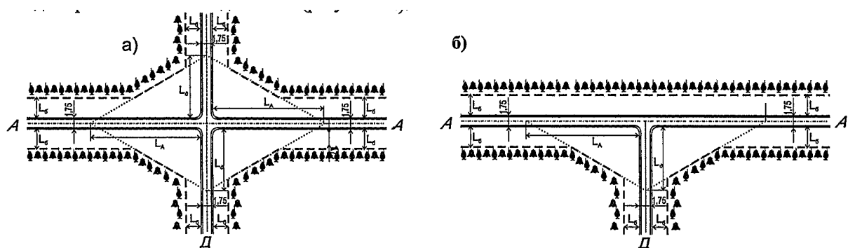
а – на пересечениях автомобильных дорог в одном уровне; б – на примыканиях автомобильных дорог в одном уровне; L_a и L_d – расстояние видимости поверхности дороги; L_b – расстояние боковой видимости; граница зоны видимости показана пунктиром
