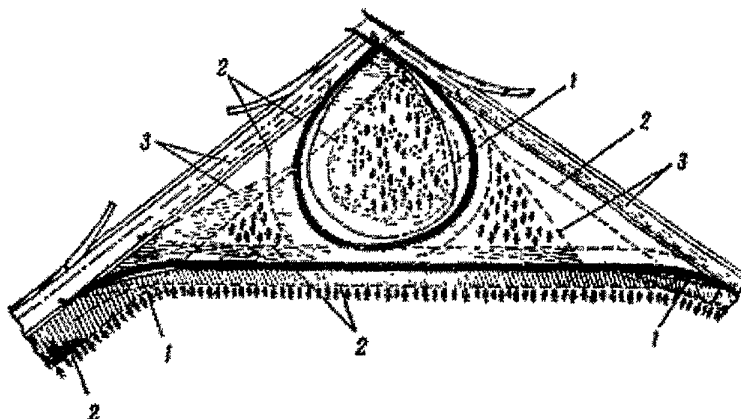
1 – границы зоны видимости внутри кривых; 2 – границы зоны боковой видимости; 3 – границы зоны видимости на въездах со съездов на магистраль
