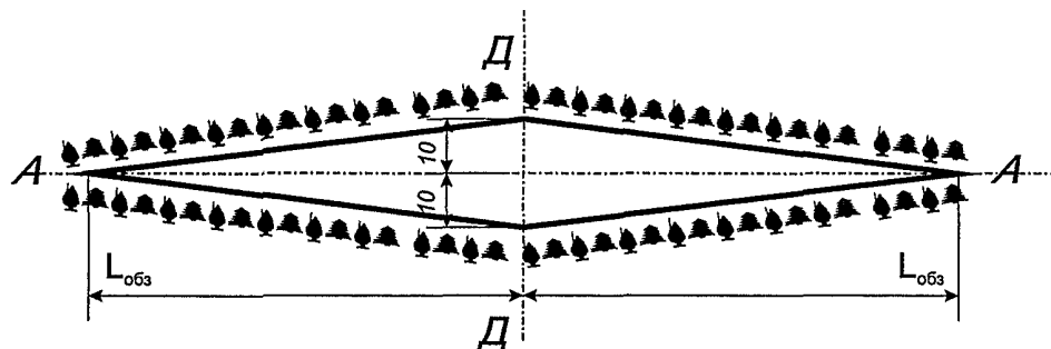
Рисунок 6.3 – Схема видимости по главной дороге и обзорности с второстепенной дорогой
