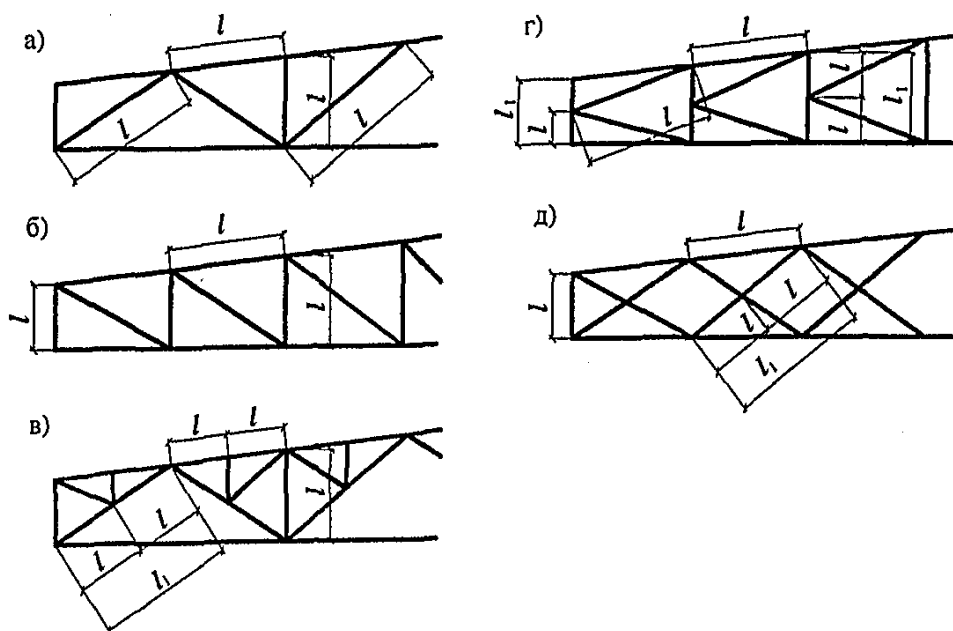
а – треугольная со стойками; б – раскосная; в – треугольная со шпренгелями; г – полураскосная треугольная; д – перекрестная
