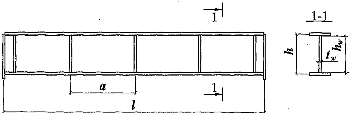
Рисунок М.1 — Схема балки с гибкой стенкой
