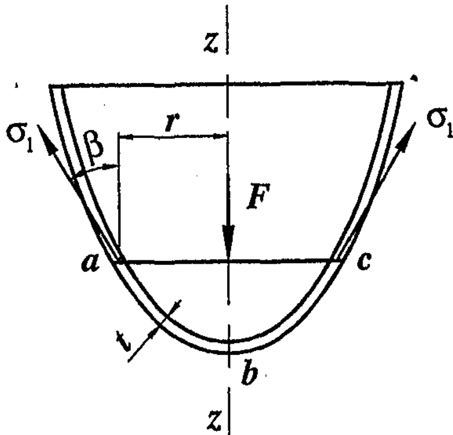
Рисунок 16 – Схема оболочки вращения
