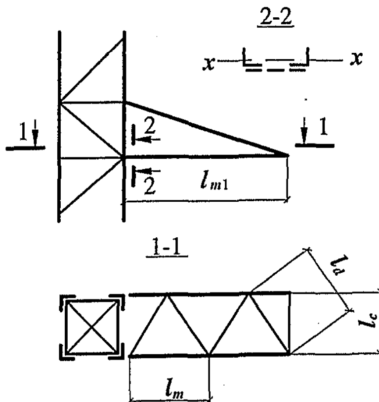
Рисунок 22 – Схема траверсы с треугольной решеткой
