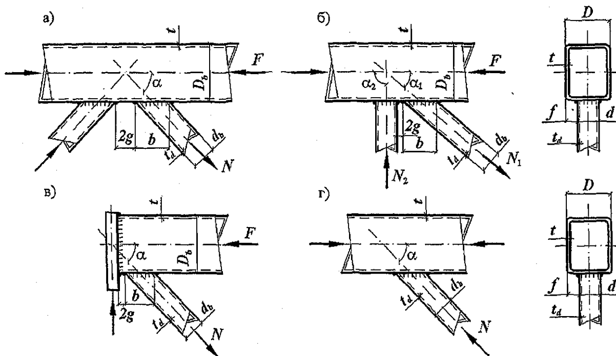
\alpha – К-образный при треугольной решетке; \beta – то же, при раскосной решетке; \sigma – опорный; \gamma – Y-образный
