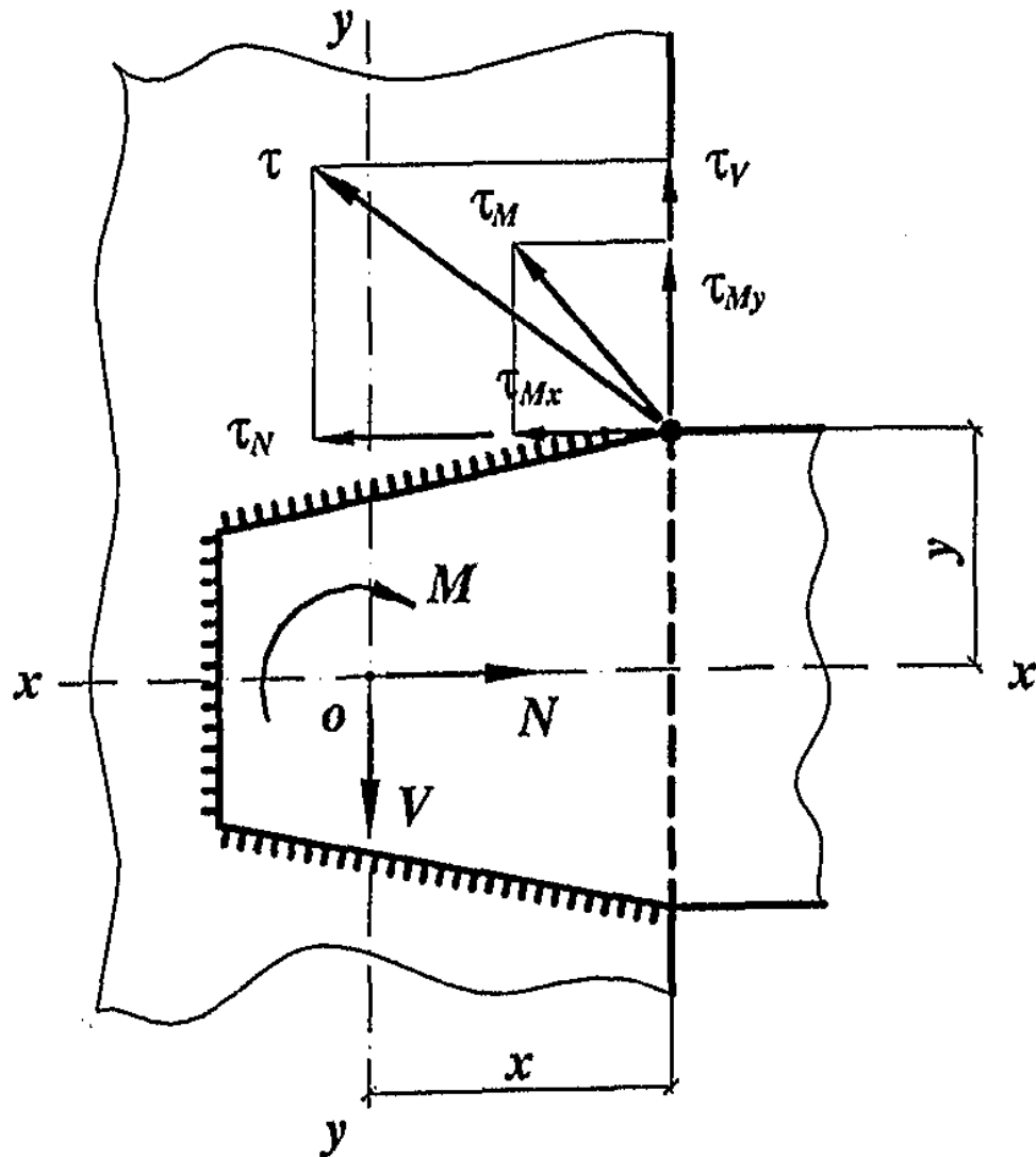
Рисунок 21 – Расчетная схема сварного соединения
