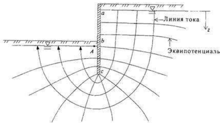
Рисунок 9.3 - Фильтрация в котлован при несовершенной ПФЗ
