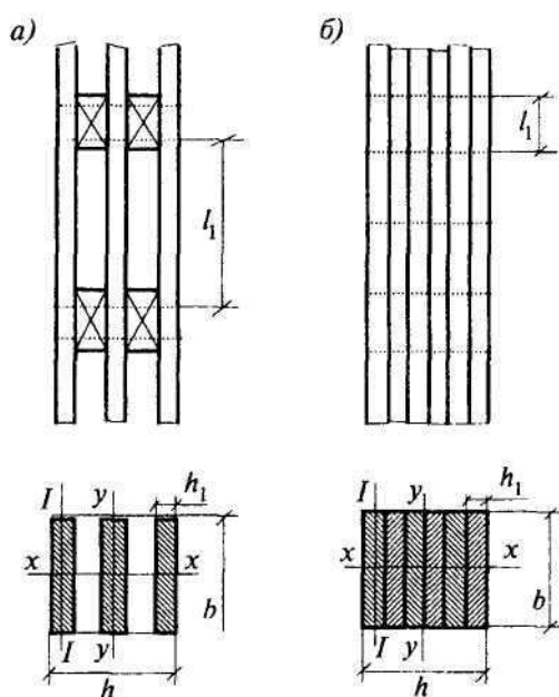
а - с прокладками; б - без прокладок
