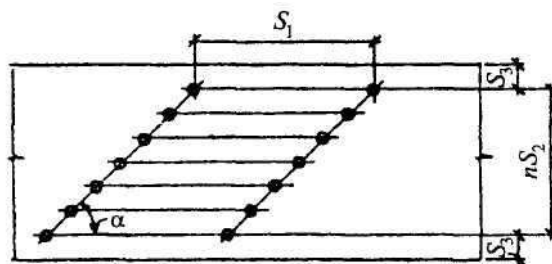
Рисунок 12 - Расстановка гвоздей косыми рядами
