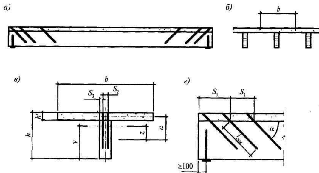
a - общий вид; б - поперечное сечение; в - геометрические характеристики поперечного сечения; г - опорная зона балки
