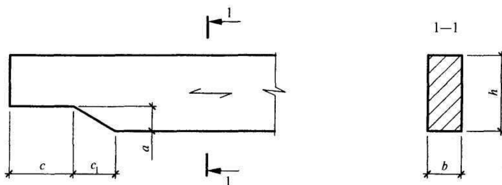
Рисунок 15 - Скошенная подрезка конца балки
