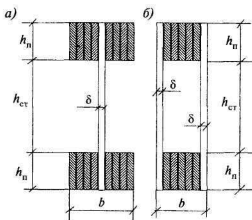
а - двутавровое сечение; б - коробчатое сечение
