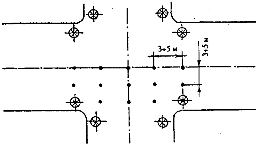
Рисунок А8 — Расположение контрольных точек при измерении средней освещенности улиц при осевом двухрядном расположении светильников
